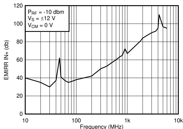
Figure 7-6. OPA2140 EMIRR
